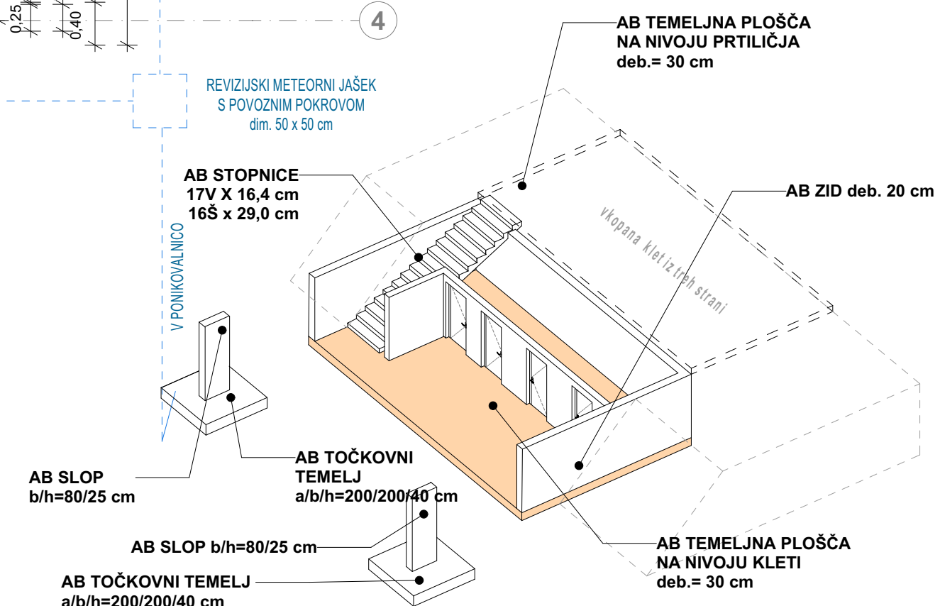
SHEMA NOSILNE KONSTRUKCIJE V KLETI (m 1:150):
