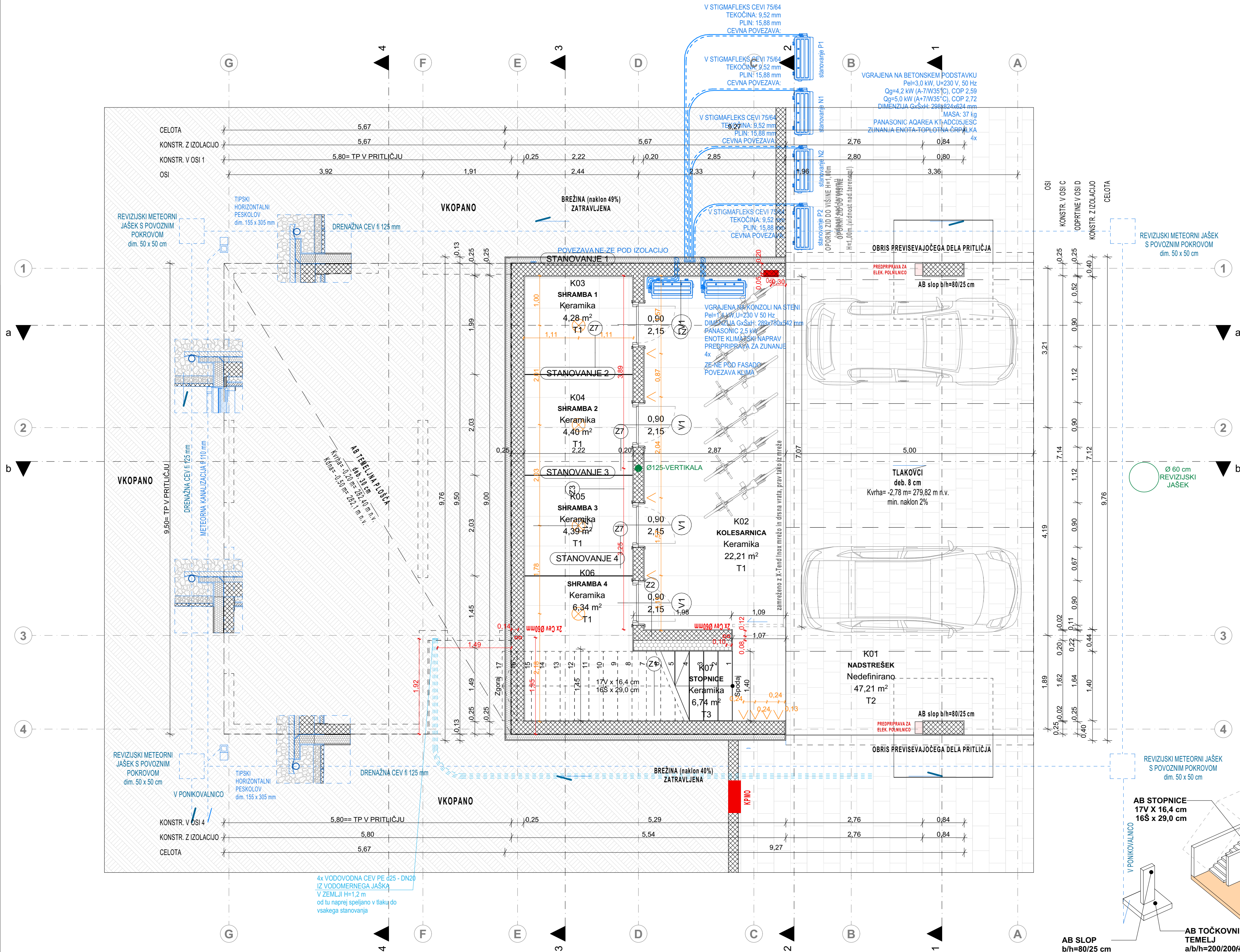
SHEMA NOSILNE KONSTRUKCIJE V KLETI (m 1:150):
