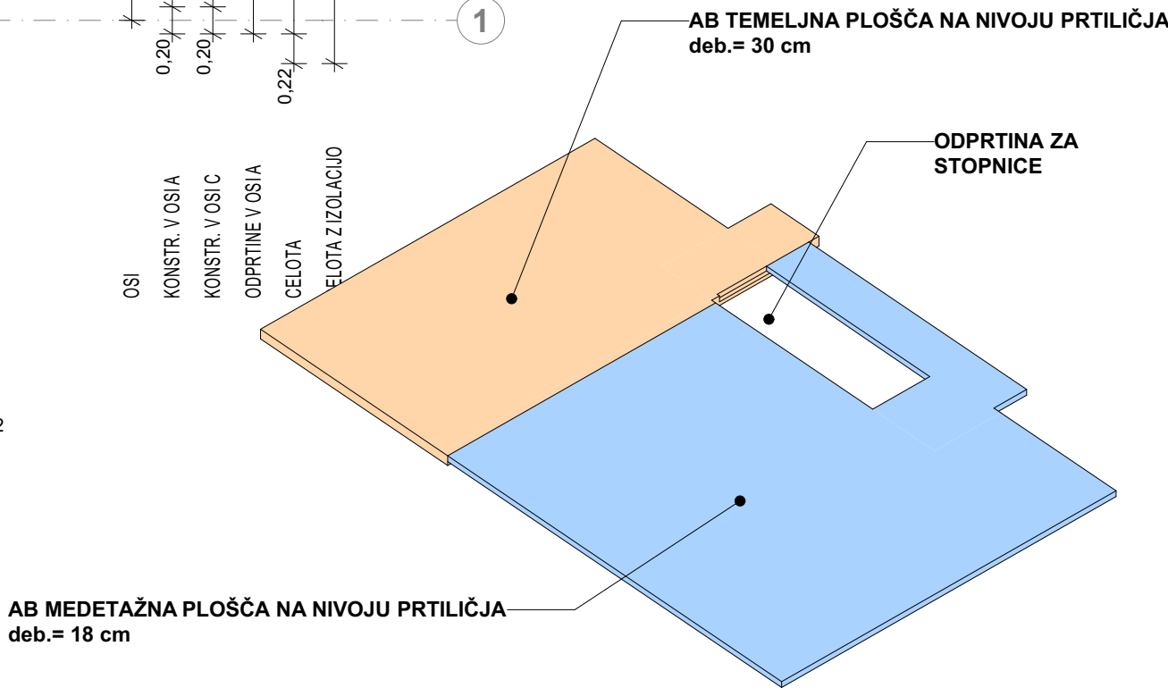
HEMA AB PLOŠČ NA NIVOJU PRITLIČJA (m 1:150):
