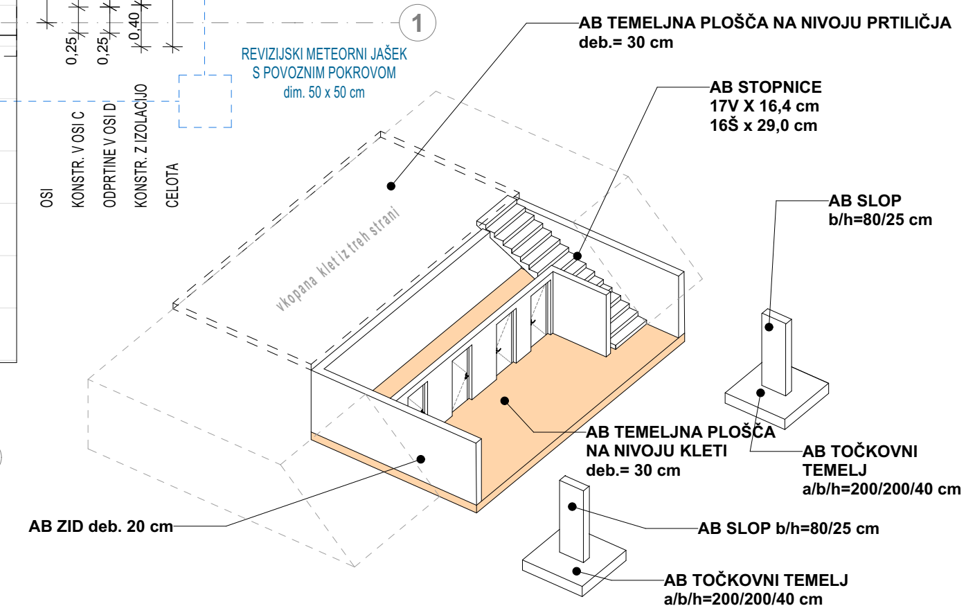
SHEMA NOSILNE KONSTRUKCIJE V KLETI (m 1:150):
